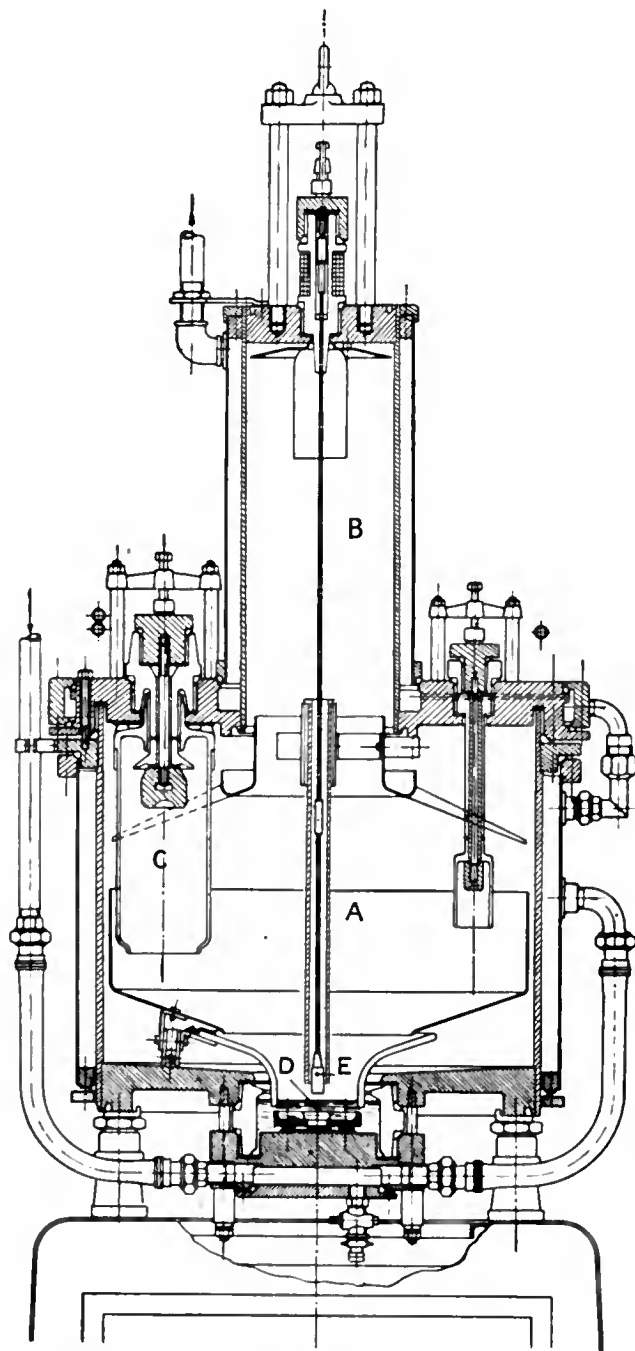
FIG. 2.—300-Ampere Mercury-Vapour Rectifier.
