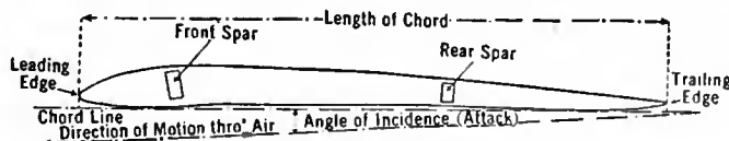
FIG. 6.—Wing Section R.A.F. 15.
